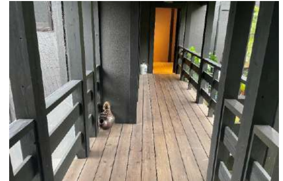
通路幅120cm
